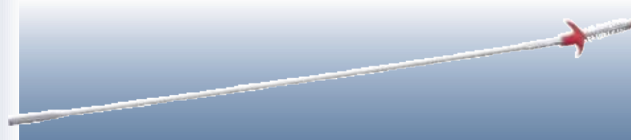
D39669 ГИБКИЙ КЛЕЩЕВОЙ ЗАХВАТ Оснащен клещевым наконечником, управляемым с помощью ручки с пружинным механизмом. Применяется для захвата небольших металлических и неметаллических предметов, попавших в труднодоступные места. Длина 610 мм. Прозрачная упаковка.
