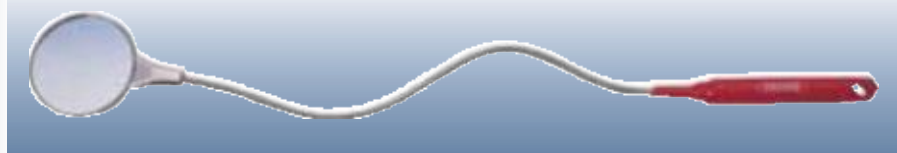
D11954 СМОТРОВОЕ ЗЕРКАЛО С ГИБКОЙ РУЧКОЙ Зеркало закреплено на гибкой ручке. Обеспечивает хороший просмотр скрытых зон. Пластиковая рукоятка. Диаметр зеркала 55 мм. Длина 470 мм. Металлизированное покрытие. Прозрачная упаковка.
