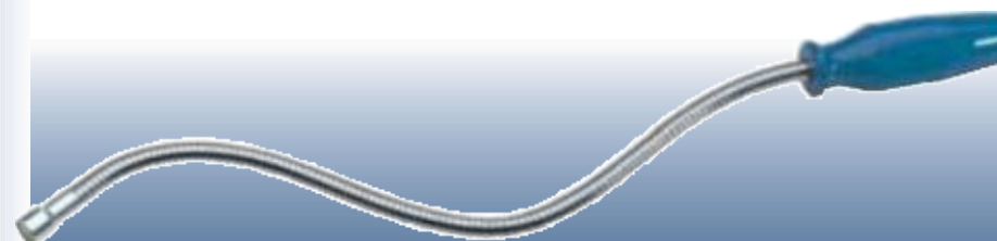
D66198 ГИБКИЙ МАГНИТНЫЙ ЗАХВАТ ПОВЫШЕННОЙ МОЩНОСТИ Профессиональное качество. Захват состоит из гибкого хромированного стержня с магнитным наконечником и пластиковой рукоятки. Поднимающая способность приблизительно 1,5 кг. Длина 540 мм. Упаковка прозрачная.
